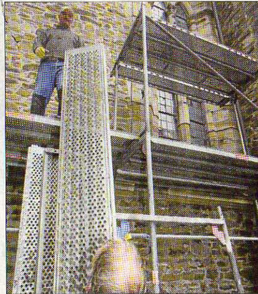
Gerüstbauer reichen Stangen und Laufplanken hinauf. Fast die halbe St.-Salvatoris-Kirche, von der Glockenstube über die Eingangsnordseite bis zum Calvör-Zimmer, wird eingerüstet. Fotos: Bertram
